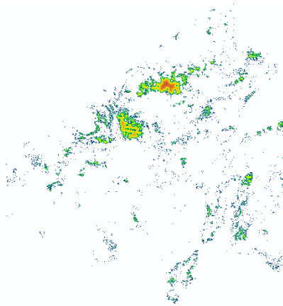
edge distance
